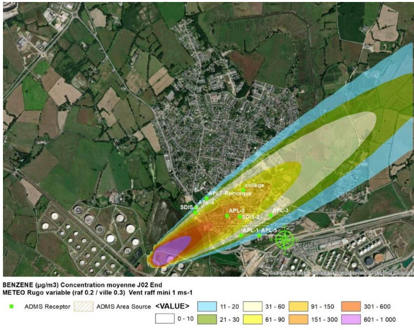
Figure 22 : simulation concentration benzène moyenne J02 de l'ordre de 10 g/s
