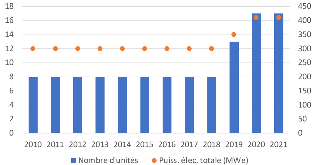
Evolution du parc de méthanisation d'industrie Valorisation en cogénération
