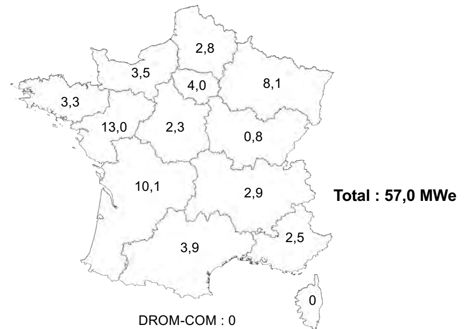
Répartition géographique des installations cogénération (en puissance installée - MWe)
